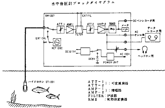
図1 原図：1977.9（沖興）2.B（水中音圧計），沖電気
