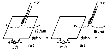
図1 図形入力装置の原理
