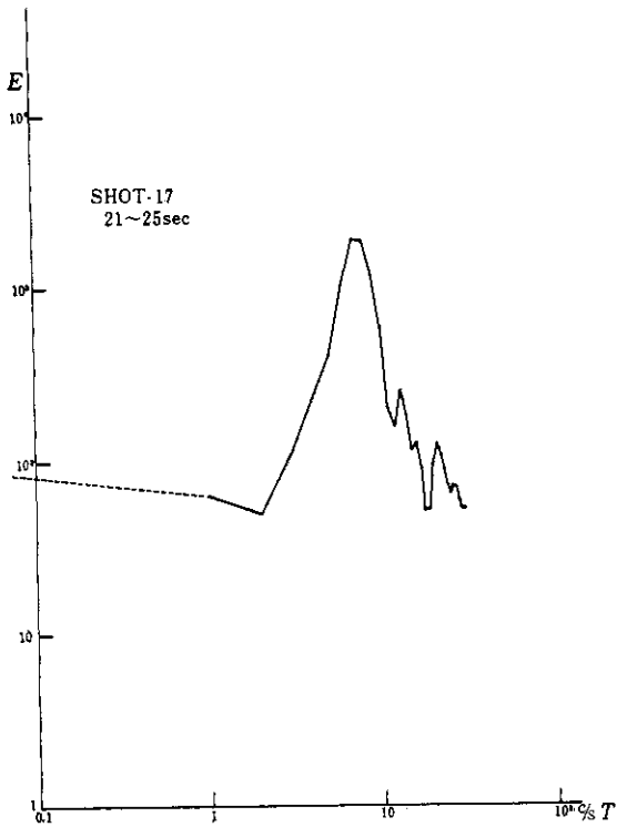
図-7-17-5 5秒ごとの周波数分析
