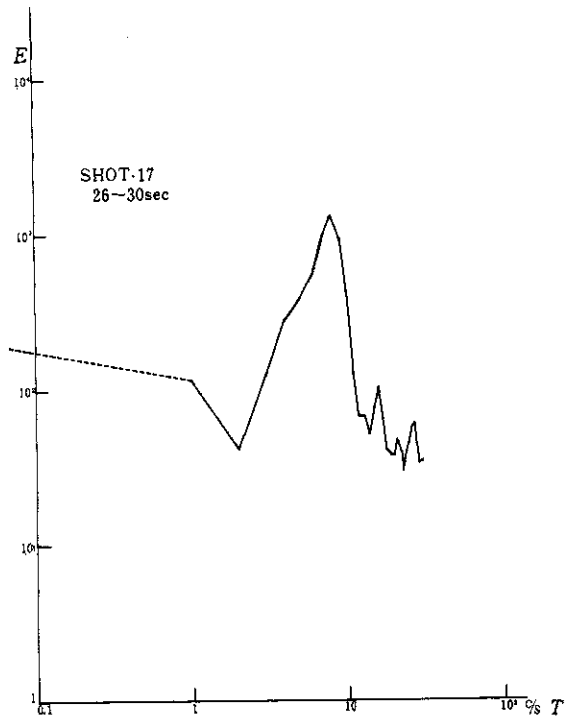
図-7-17-6 5秒ごとの周波数分析
