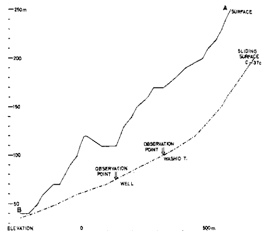
図-5 炭層C37cの断面図(図-6のA-B)
