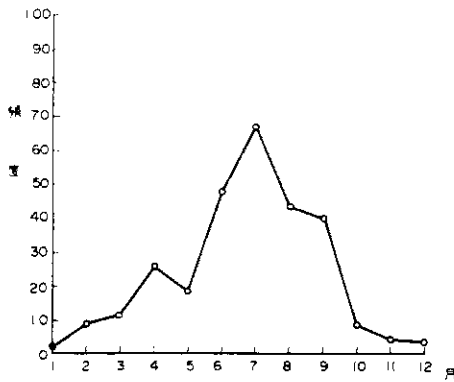
図-7 佐世保市における日降水量10mm以上が1日間隔で発生する頻度の季節変化
