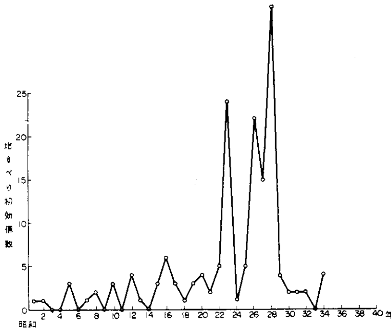
図-1 長崎県における地すべり初効個数の年次変動
