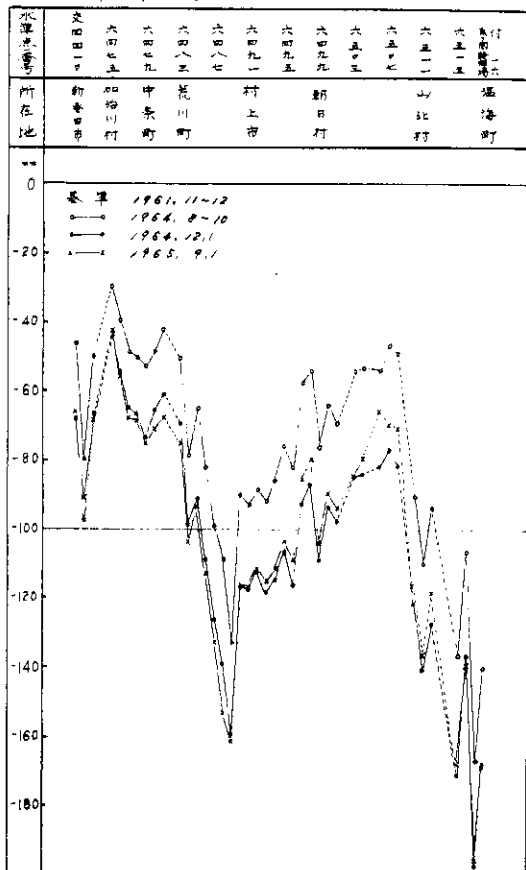
図-2 地震およびその後の水準点上下変動。柏崎水準点No.3742を不動点と仮定。
