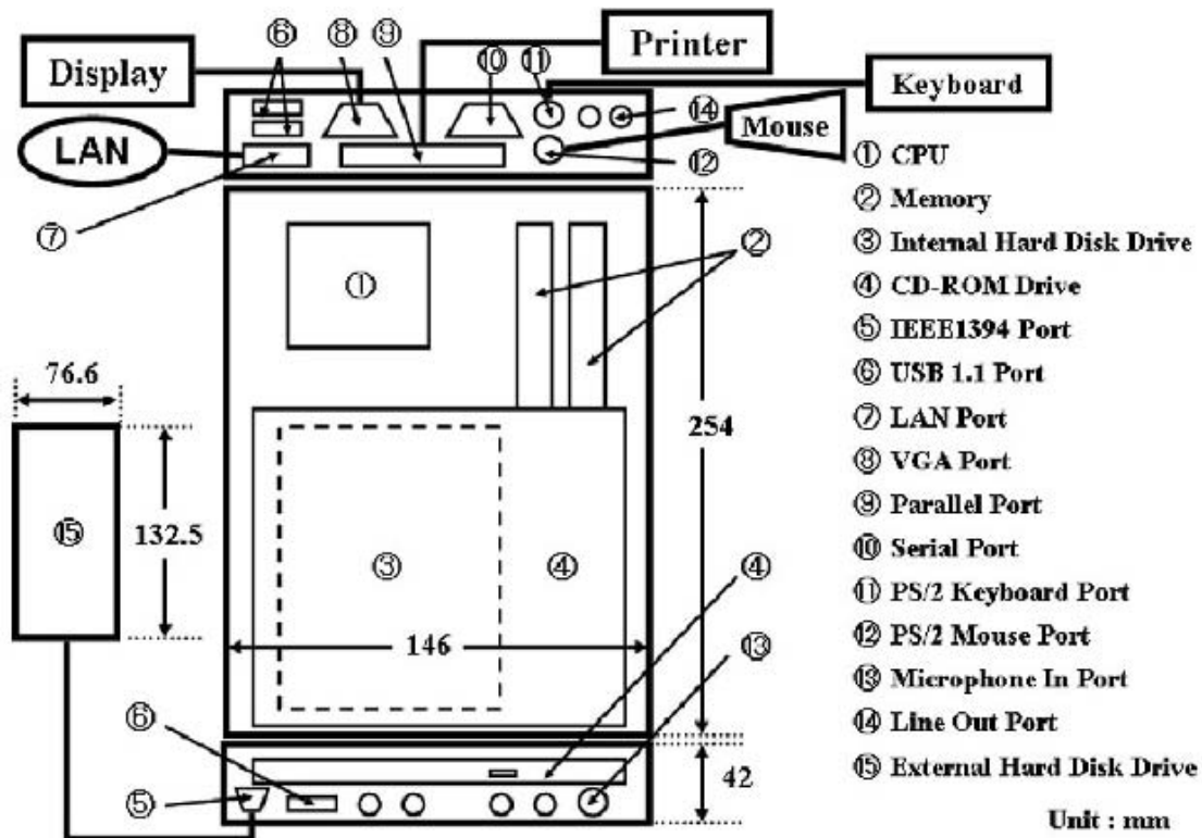
図3 システム図 Fig. 3 System configuration.
