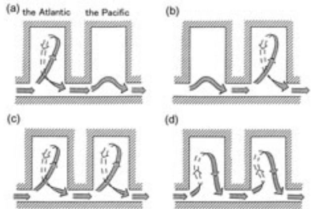
図 2 海洋の深層循環の同一境界条件下の多重解の例 (Held, 1993 による Marotzke and Willebrand, 1991 の解説から)。同一境界条件下で現在の循環のパターン (a) のほかに少なくとも 3 つの (b, c, d) パターンが存在する。それぞれのパターンに応じて気候の状態は大きく変わる。
