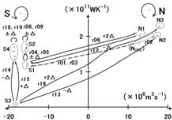
図 6 海洋の深層循環のパターンの遷移についての数値実験結果の概要。縦軸 ( \dot{S} ) はエントロピー生成率 ( \text{W K}^{-1} )、横軸 ( \Psi ) は流線関数の最大値（つまり、循環の強さ、 \text{SV}=10^6 \text{ m}^3 \text{ s}^{-1} ）を表す。左側にある点は南沈込の循環をもつ解（S の頭文字で示す）、右側にある点は北沈込の循環をもつ解（N の頭文字で示す）、矢印は遷移の方向、矢印の横にある記号は実験番号と遷移のためのトリガーとして与えた擾乱の大きさと符号を表す（例：r04 と \Delta ）。
